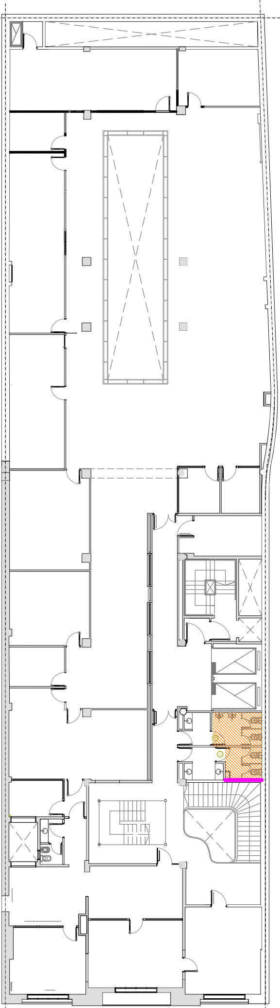
PLANTA 2° PISO
