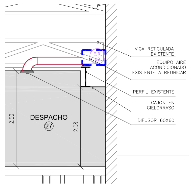
DETALLE A
