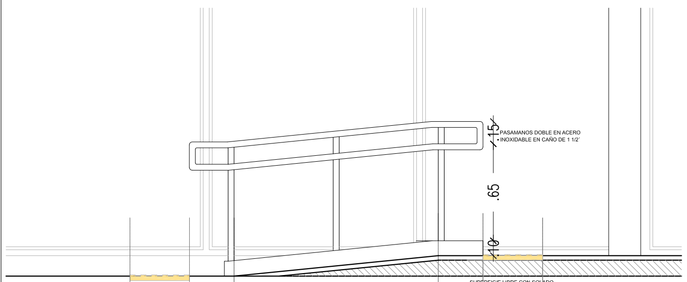
CORTE B-B
