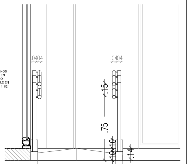
CORTE A-A
