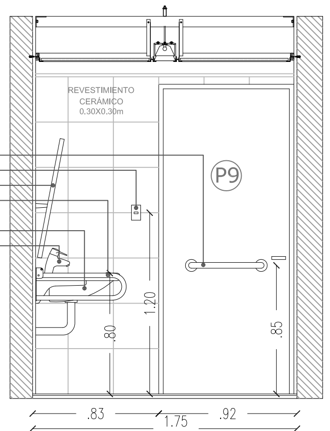
CORTE D-D
