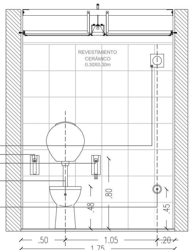
CORTE C-C
