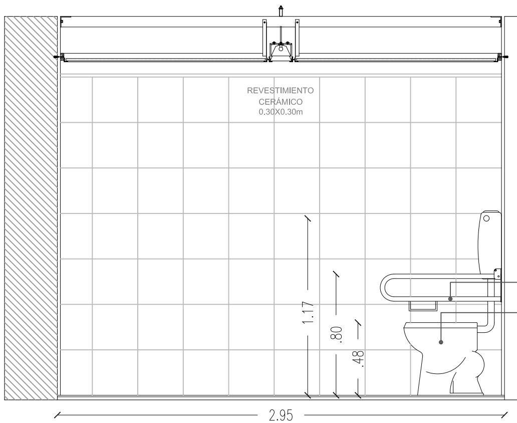
CORTE A-A
