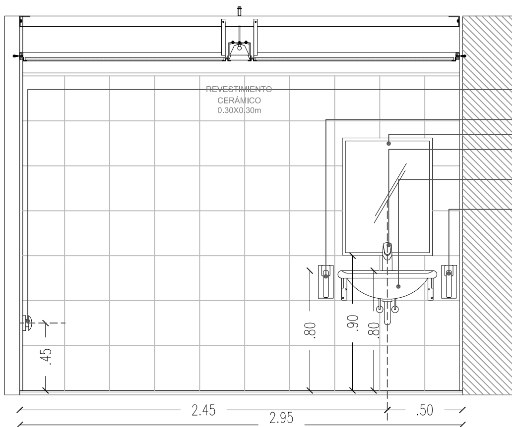
CORTE B-B
