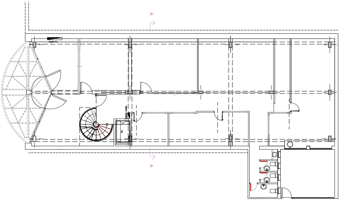
PLANTA BAJA
