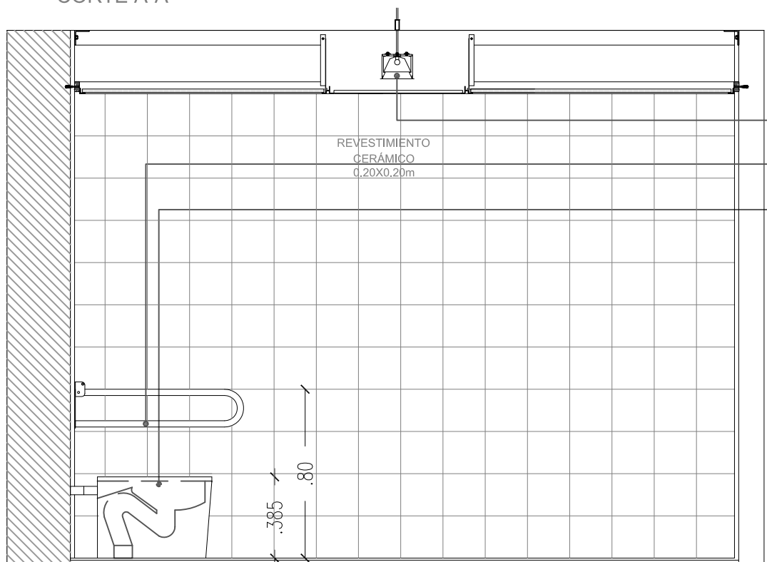
CORTE A-A
