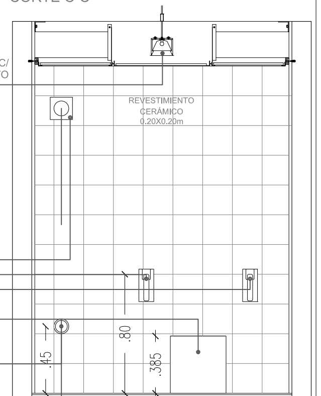
CORTE C-C
