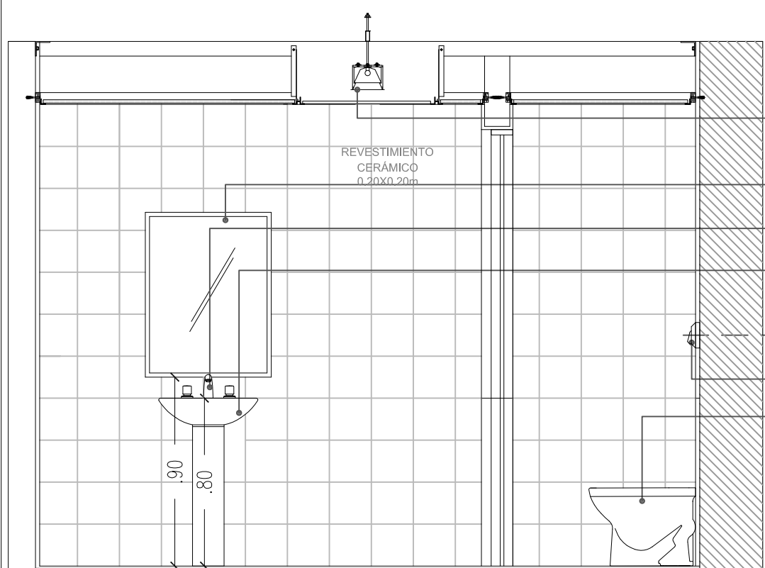
CORTE A-A
