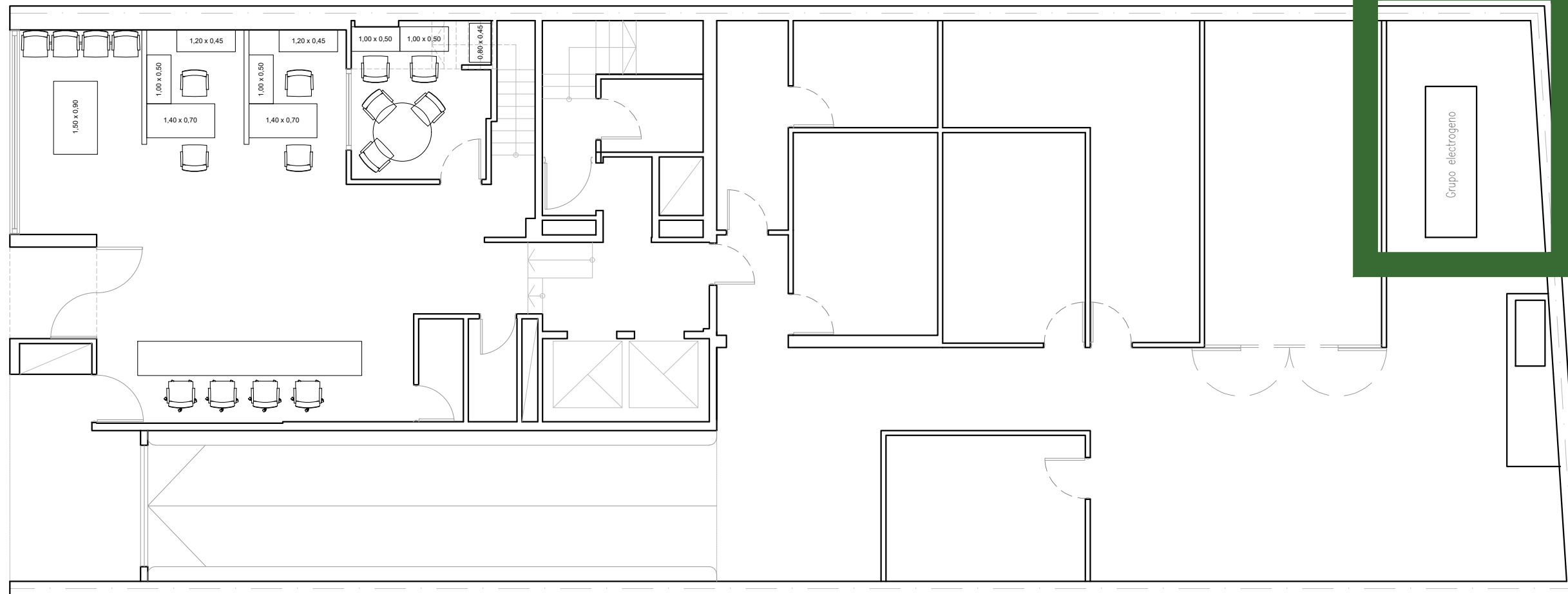
Planta Baja
